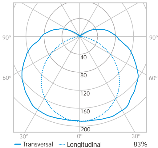
Curva de Distribuição Luminosa (cd/1000 lm)
