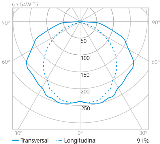
Curva de Distribuição Luminosa (cd/1000 lm)
